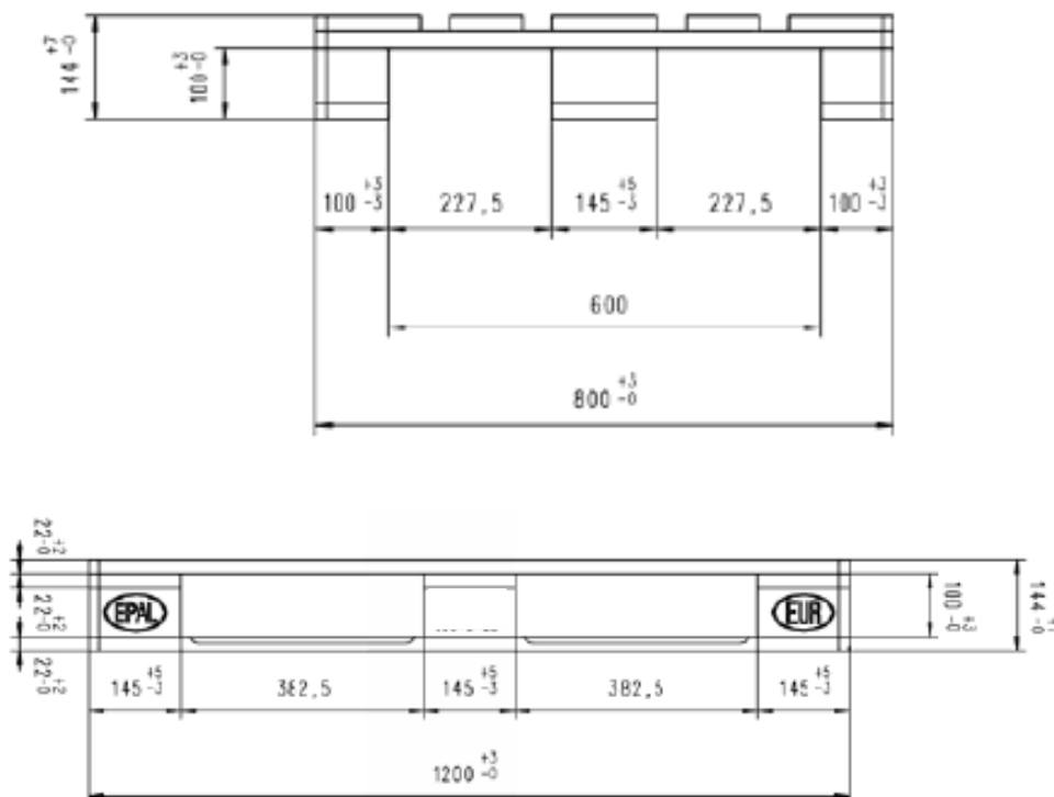
Abbildung 3: Matoleranzen gem UIC 435-2
